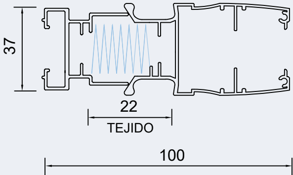
Mosquitera Cerrada: Perfil Fijo + Perfil Móvil
