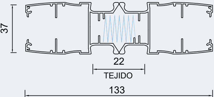
Mosquitera Cerrada: Perfil Fijo + Perfil Móvil
